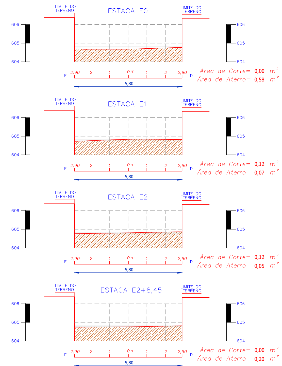
SEÇÕES TRANSVERSAIS ESCALA 1/100
