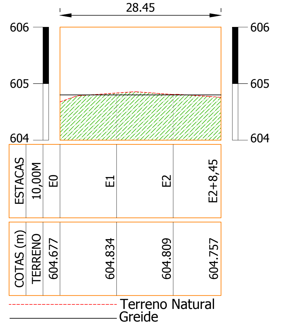
PERFIL LONGITUDINAL ESCALA 1/400
